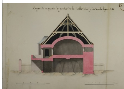
Plan et coupe de la Noble Tour, état en 1815. Le premier niveau, édifié en 1402, est complètement comblé et n'apparaît pas sur ce document, le deuxième niveau (1403) n'est visible qu'en partie. Le troisième niveau et le comble sont nettement plus récents. © AD Nord, 56Fi495bis, cliché et montage Ch. Cerci - Inrap.
