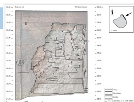
Élévation de la face nord-ouest de la Noble Tour. © Infographie et interprétation E. Delmont, photogrammétrie F. Audouit - Inrap.
